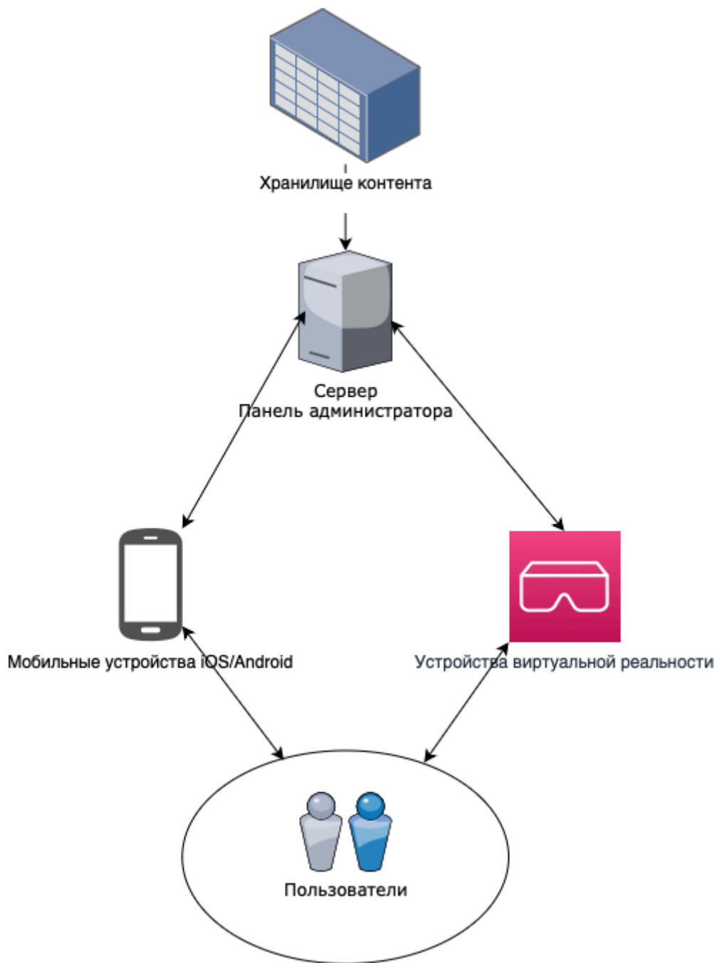
Архитектура ПО "Altairika"
